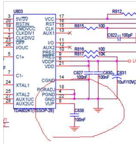
그림 5. 변형된 회로도 Fig. 5. Modified circuit
